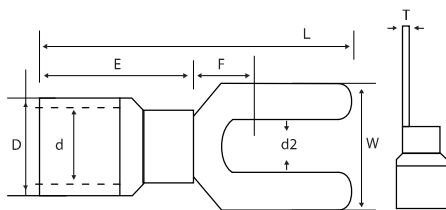
Διαστάσεις (mm)
