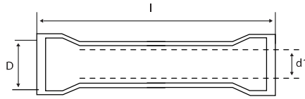
Διαστάσεις (mm)
