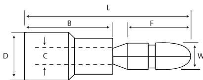
Διαστάσεις (mm)
