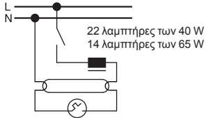
Επαγωγικό (Χωρίς αντιστάθμιση)
