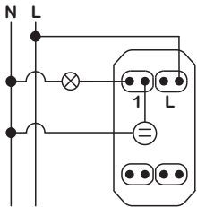
Απλή σύνδεση
