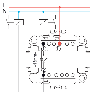
2 διακόπτες αλέ-ρετούρ με λυχνίες προσανατολισμού
