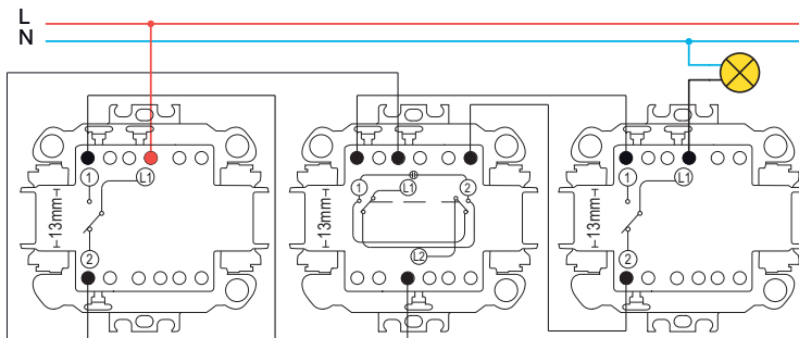
2 διακόπτες αλέ-ρετούρ + 1 μεσαίος αλέ-ρετούρ
