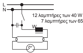
Παράλληλη αντιστάθμιση
