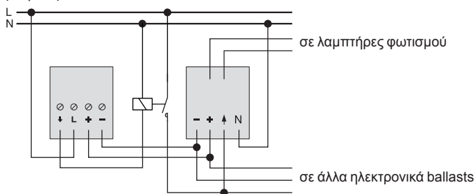
Διάγραμμα σύνδεσης μηχανισμού ρυθμιστή λαμπτήρων φθορισμού, με ηλεκτρονικά ballasts
