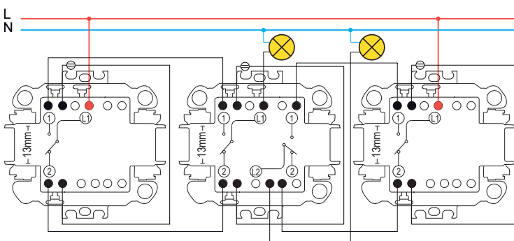
2 διακόπτες αλέ-ρετούρ + 1 διακόπτης διπλός αλέ-ρετούρ
