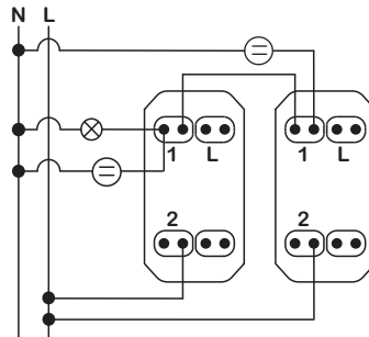
Αλέ-ρετούρ σύνδεση
