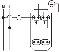
Απλή σύνδεση
