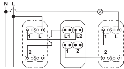
Σύνδεση αλέ-ρετούρ με ενδιάμεσο διακόπτη
