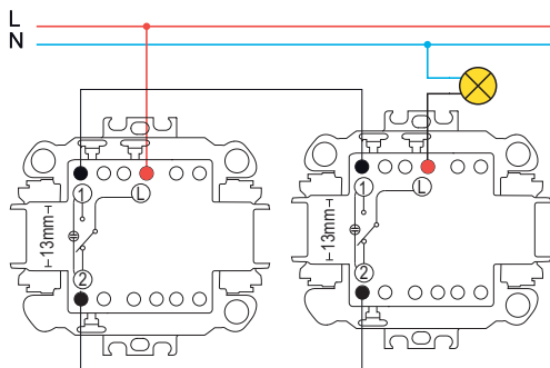
2 διακόπτες αλέ-ρετούρ
