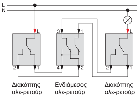
Υπάρχον κύκλωμα με ενδιάμεσο αλέ-ρετούρ
