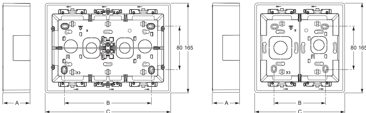
Οριζόντια Κουτιά
