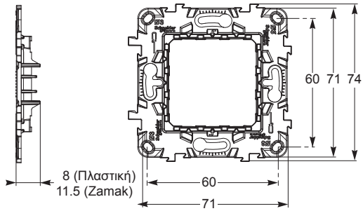
Zamak και πλαστική (2 στοιχεία)
