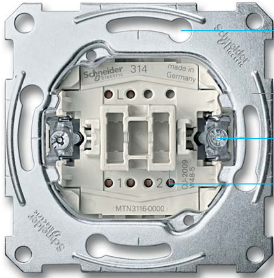
Χωνευτός μηχανισμός διακόπτη QuickFlex®
