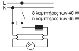
Παράλληλη αντιστάθμιση
