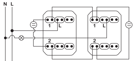
Σύνδεση αλέ-ρετούρ
