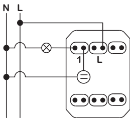
Απλή σύνδεση
