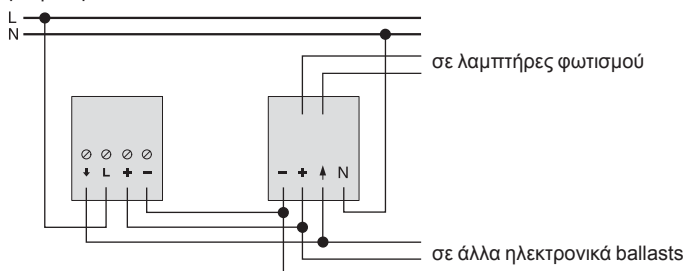
Διάγραμμα σύνδεσης μηχανισμού ρυθμιστή λαμπτήρων φθορισμού, με ηλεκτρονικά ballasts
