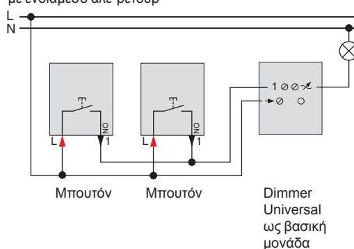
Ρύθμιση έντασης φωτισμού σε κύκλωμα με ενδιάμεσο αλέ-ρετούρ
