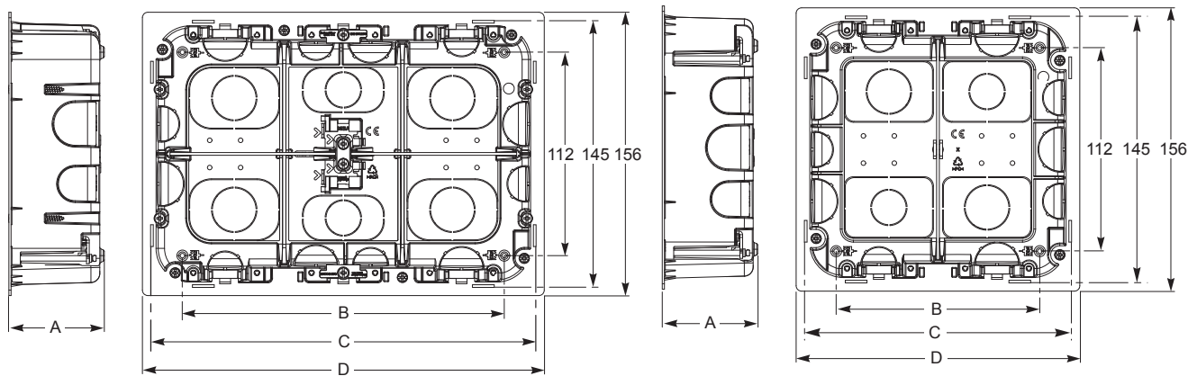
Οριζόντια κουτιά
