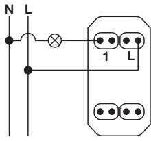
Απλή σύνδεση
