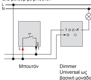
Ρύθμιση έντασης φωτισμού σε κύκλωμα αλέ-ρετούρ με μπουτόν
