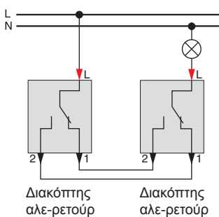
Υπάρχον κύκλωμα αλέ-ρετούρ
