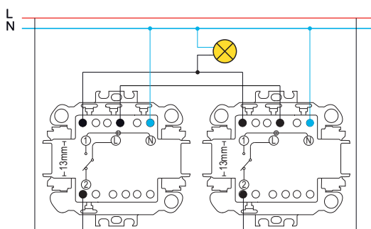
2 διακόπτες αλέ-ρετούρ
