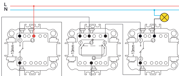
2 διακόπτες αλέ-ρετούρ + 1 μεσαίος αλέ-ρετούρ με λυχνίες προσανατολισμού
