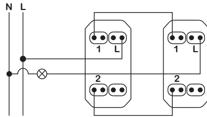
Αλέ-ρετούρ σύνδεση
