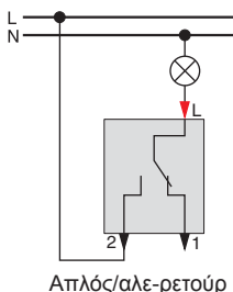
Απλός/αλέ-ρετούρ
