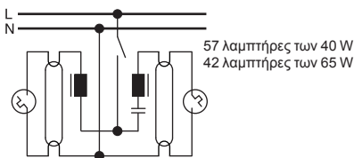
Κύκλωμα με δύο λαμπτήρες
