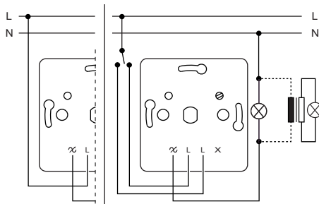
Σύνδεση αλέ-ρετούρ - EPH64001xx - EPH65001xx
