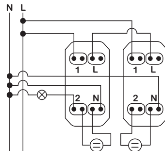
Σύνδεση αλέ-ρετούρ με ενδεικτική λυχνία και ουδέτερο
