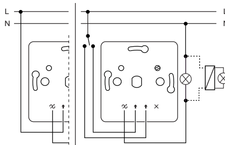
Σύνδεση αλέ-ρετούρ - EPH66001xx
