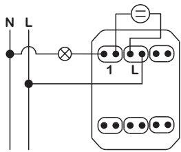
2 στοιχείων - Απλός διακόπτης με λυχνία προσανατολισμού
