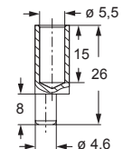
CGT 16
