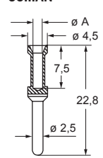
CC...AN
